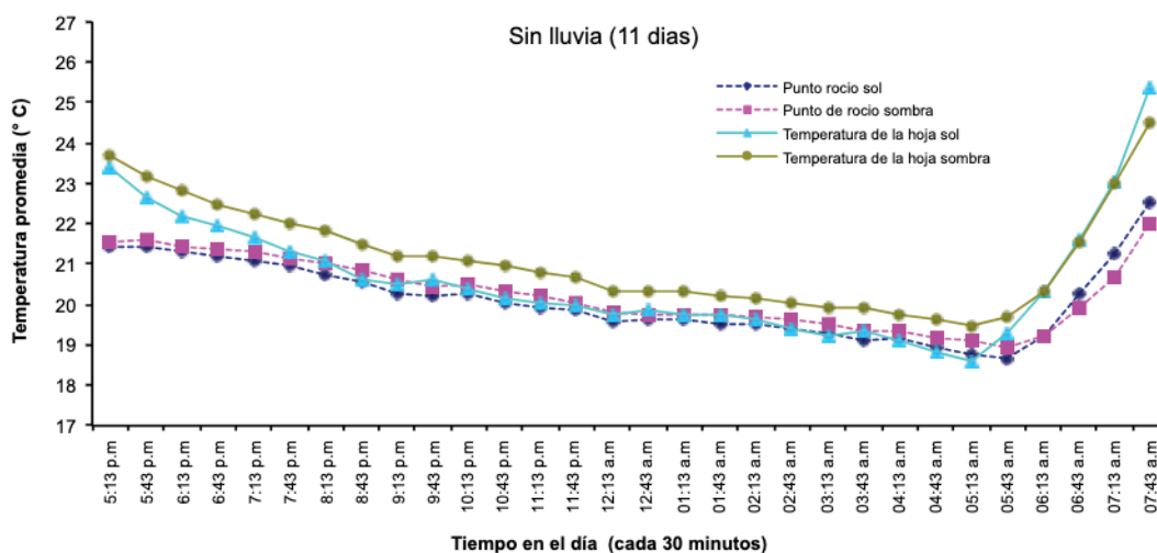
Figura 2. Comparación de la temperatura de hoja (línea continua) y el punto de rocío (línea discontinua) en condición sin lluvia, para los ensayos sol y sombra, en el periodo 2009 Fuente: López (2010).
